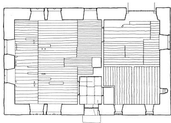
Opmåling 1986 ved byggeteknikeruddannelsen, Bornholms Erhvervsskole. Se ("Kampestensbygninger i Sandvig". 1986).
